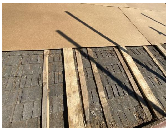
Fig. 5. Masonite läggs över det undre taket.
